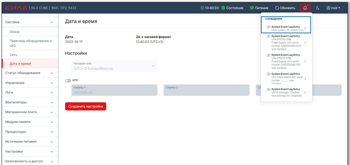
Рисунок 53. Список сообщений
