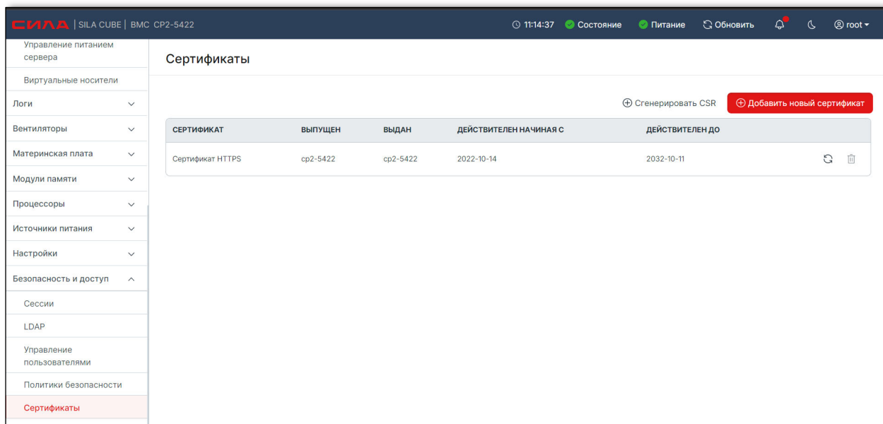
Рисунок 11. Страница «Сертификаты»
