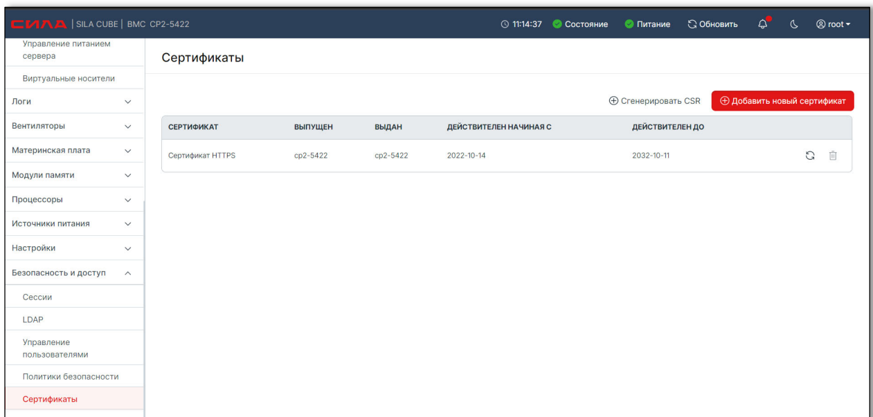
Рисунок 8. Страница «Сертификаты»
