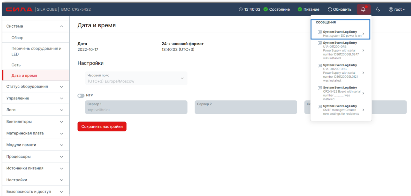
Рисунок 55. Список сообщений
