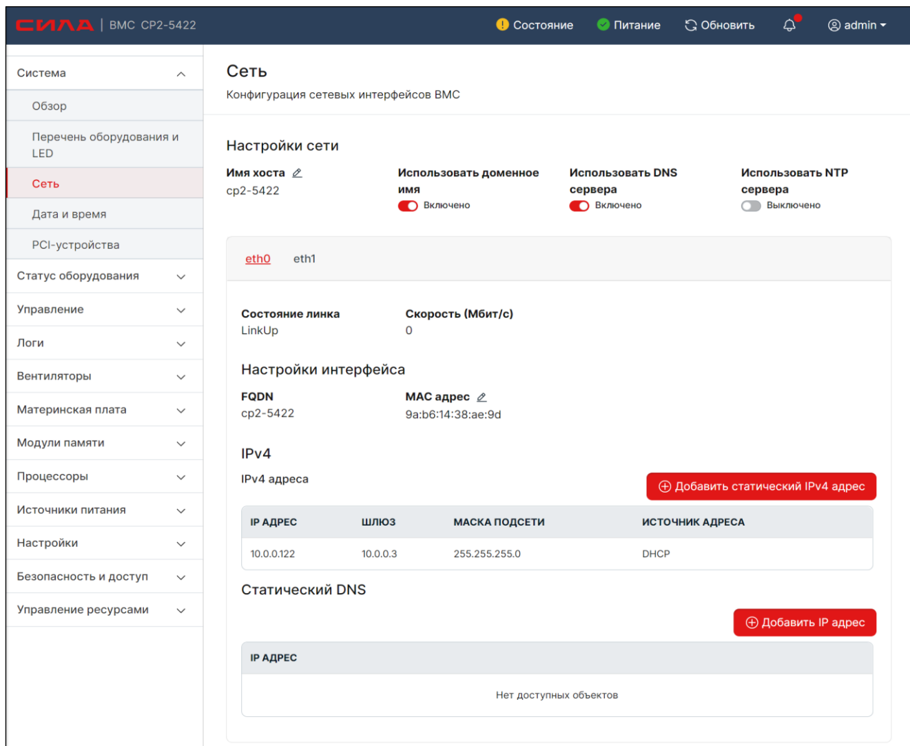
Рисунок 30. Страница «Сеть»
