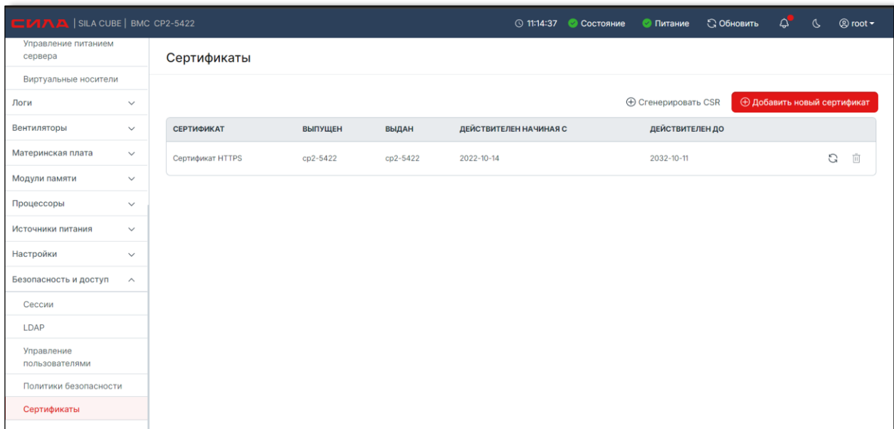
Рисунок 11. Страница «Сертификаты»
